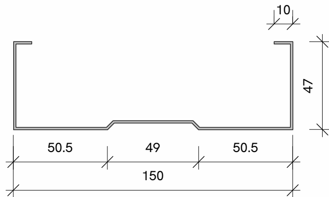
3 SEÇÃO - PERFIL 150 mm ESCALA 1 : 2
