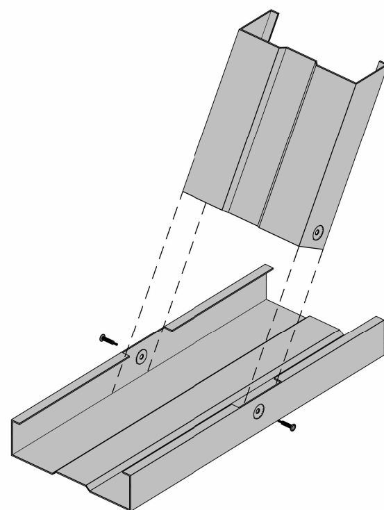
3 PERSPECTIVAS - UNIÃO PERFIL INCLINADO ESCALA
