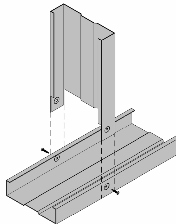
2 PERSPECTIVAS - UNIÃO ENTRE PERFIS NO MEIO ESCALA
